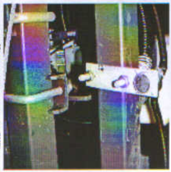
Кронштейн крепления (ШП) установленный рядом ягути.
