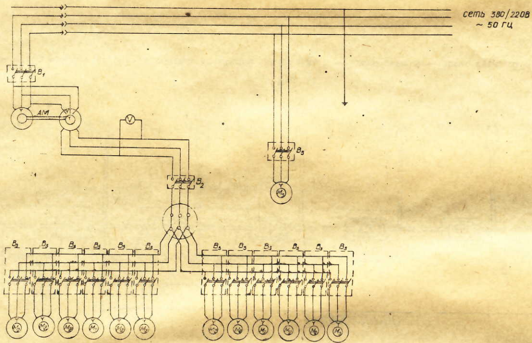
Рис. 12. Принципиальная электрическая схема агрегата ЭСА-12/200
