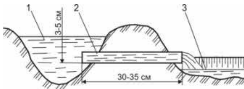
Рис. 2. Применение поливных трубок при распределении воды по бороздам
