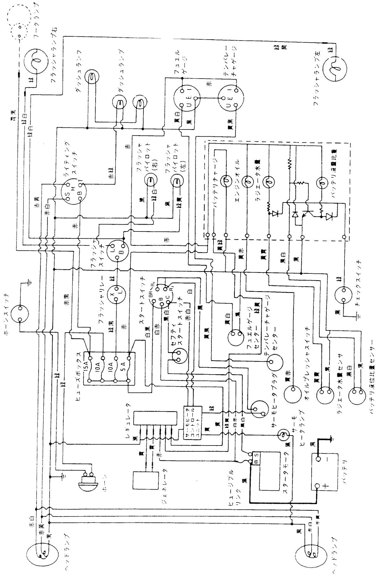
配線図
