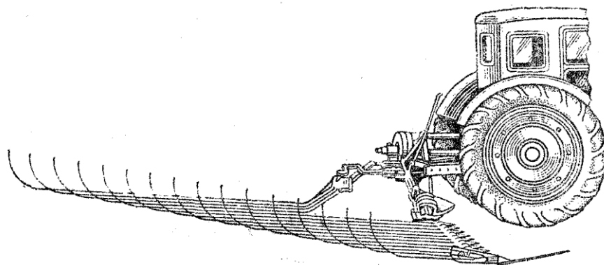
Рис. 178. Косилка КС-2,1 с приспособлением ПБ-2,1 и устройством ПБА-4 для уборки бобовых культур
