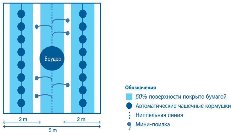
Рис. 4: Типичное размещение точечного брудера (на 1000 цыплят)
