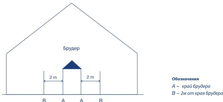
Рис. 5: Точечный брудер – температурные зоны
