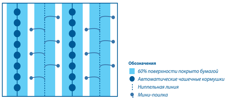
Рис. 8: Типичное устройство птичника при использовании всего помещения в брудерный период
