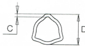
Внутренняя труба
