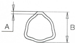
Внешняя труба
