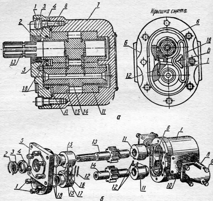
Рис. 9. Шестеренчатый насос типа НШ:
