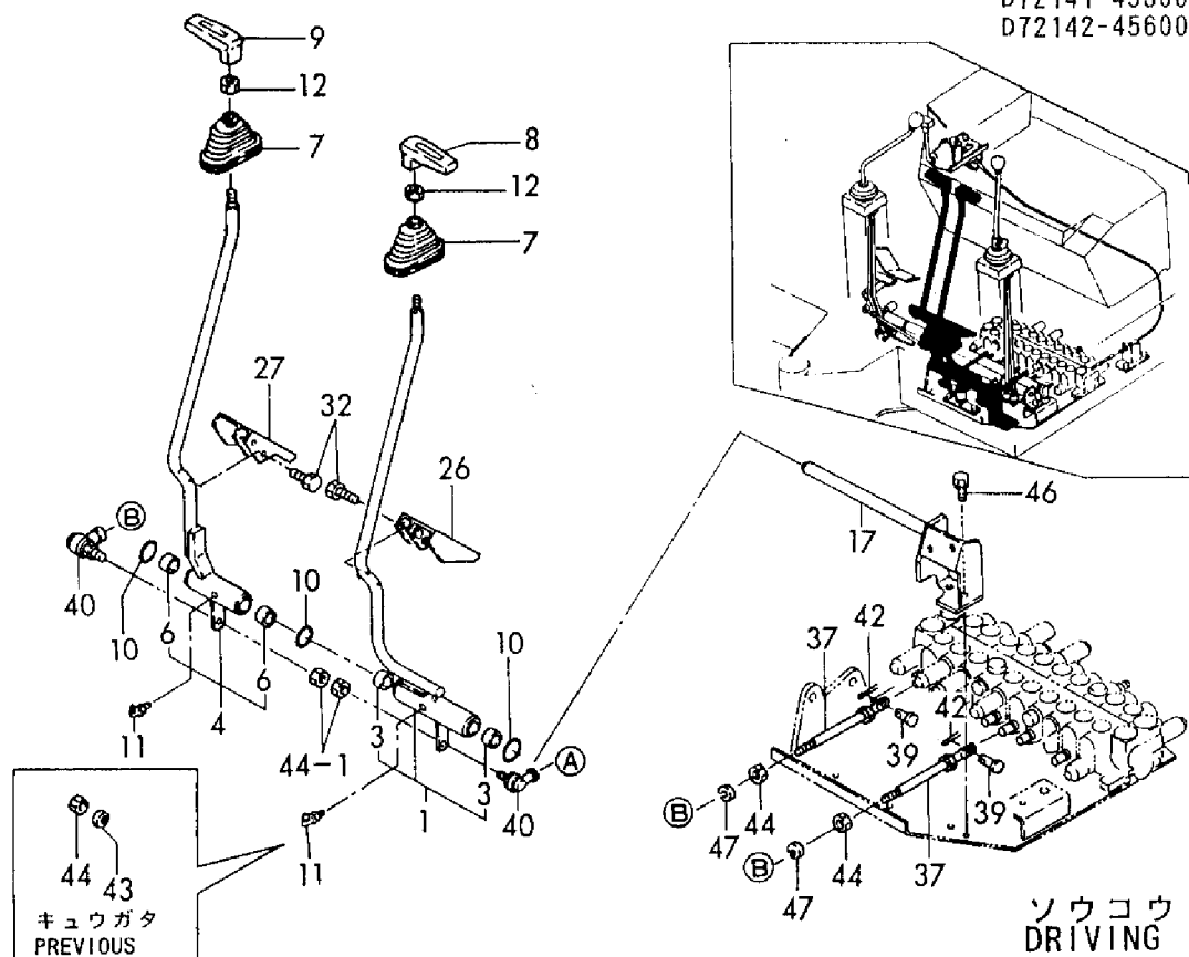
Fig. 27 ソウジュウソウチ(ソコウ & スイング) CONTROL EQUIP. (DRIVING & SWING)
