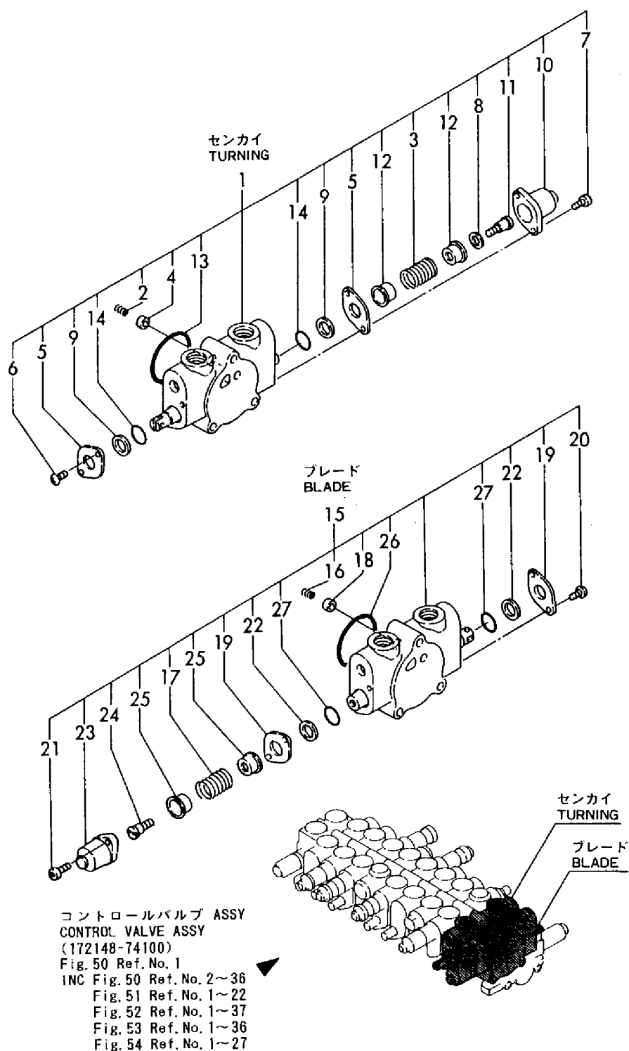
Fig. 54 コントロールバルブ(センカイ & ブレード) CONTROL VALVE(TURNING & BLADE)
