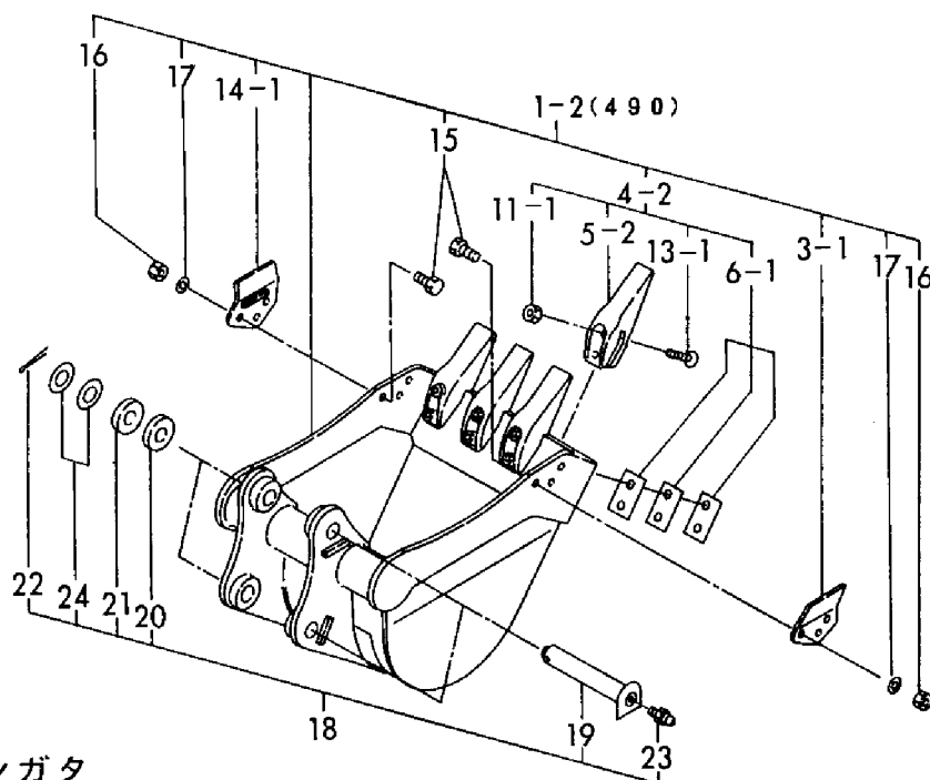
Fig. 73 バケット(450, 490)(アタッチメント) BUCKET(450, 490)(ATTACHMENT)
