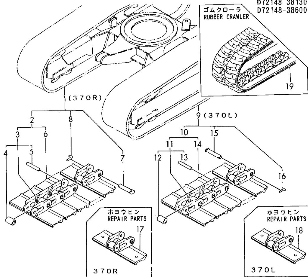
Fig. 19 クローラ CRAWLER
