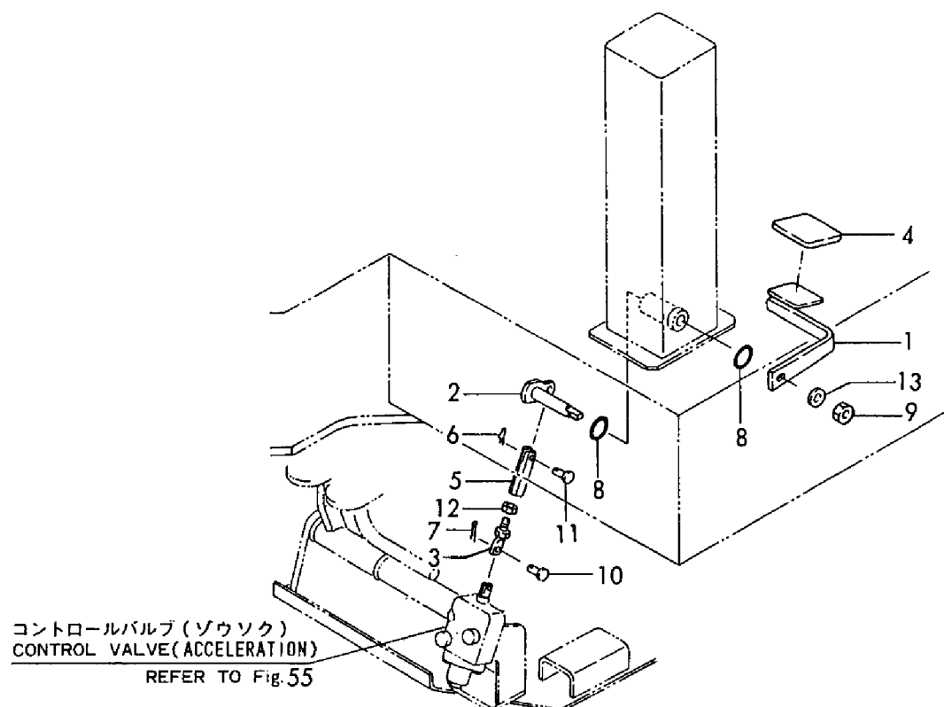
Fig. 21 ソウジュウソウチ (ゾウソクペダル) SPEC. CODE CONTROL EQUIP. (ACCELERATOR PEDAL) D72148-41700
