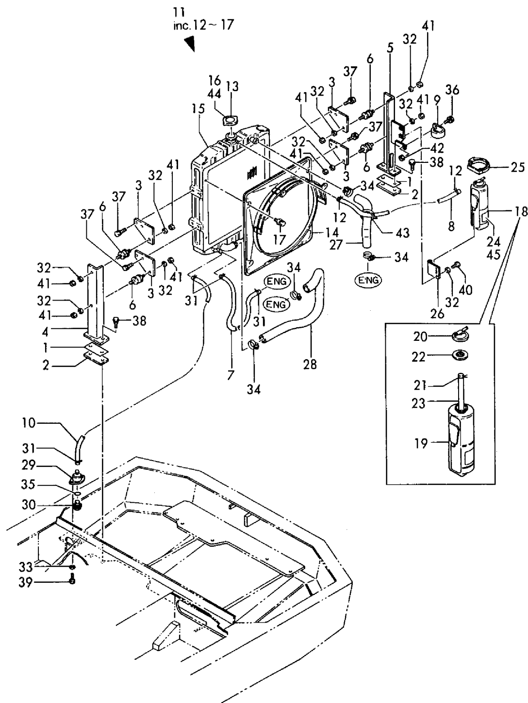
Fig. 10 ラジエータ & マウント RADIATOR & MOUNT
