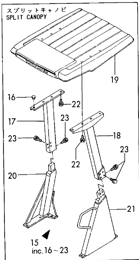
Fig. 38 キャンピ CANOPY
