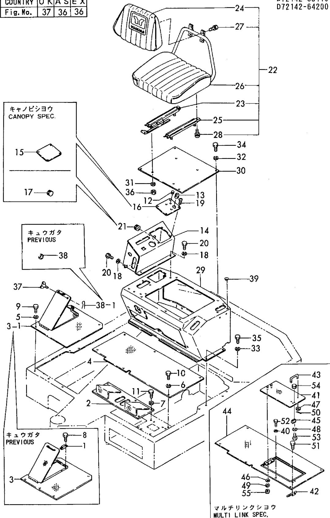
Fig. 35 シート & ステップ SEAT & STEP
