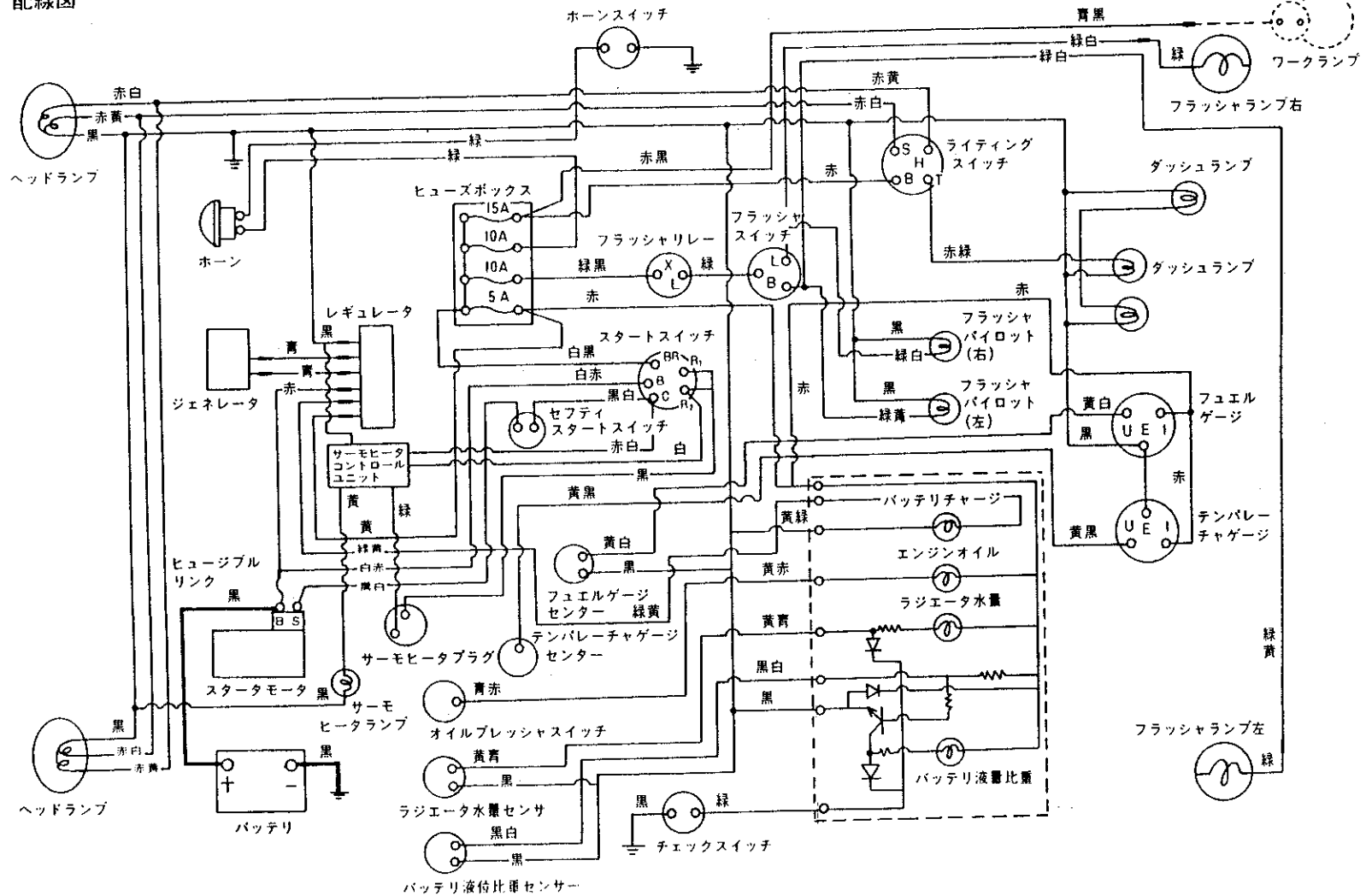
配線図
