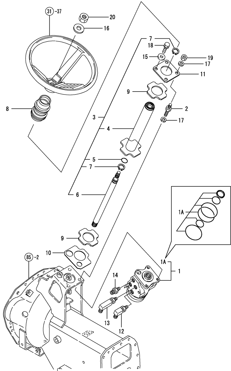
Fig.81. P.S.T VALVE(ADD.
