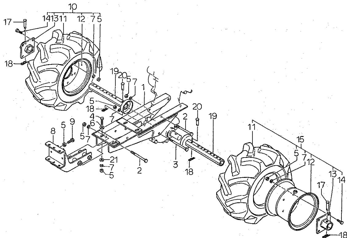
シヤシ, ホイール FIG.228 CHASSIS, WHEEL
