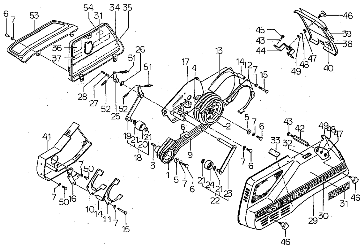
ベルト ドライブ FIG.225 BELT DRIVE
