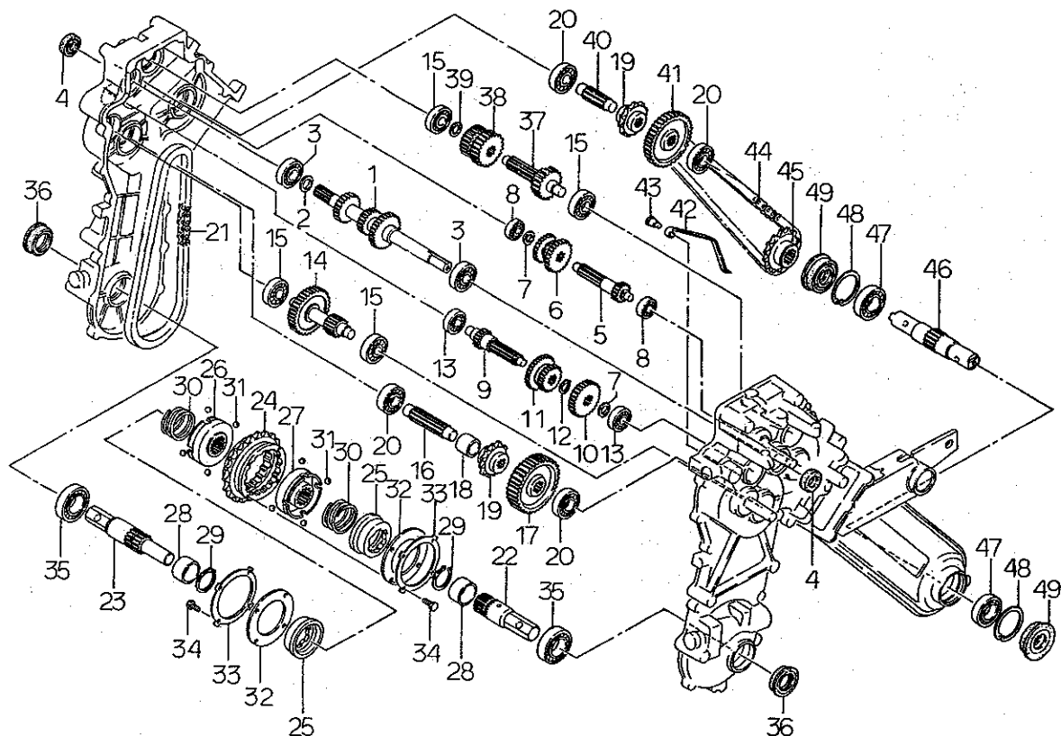
トランスミッション ギヤ FIG.222 TRANSMISSION GEARS
