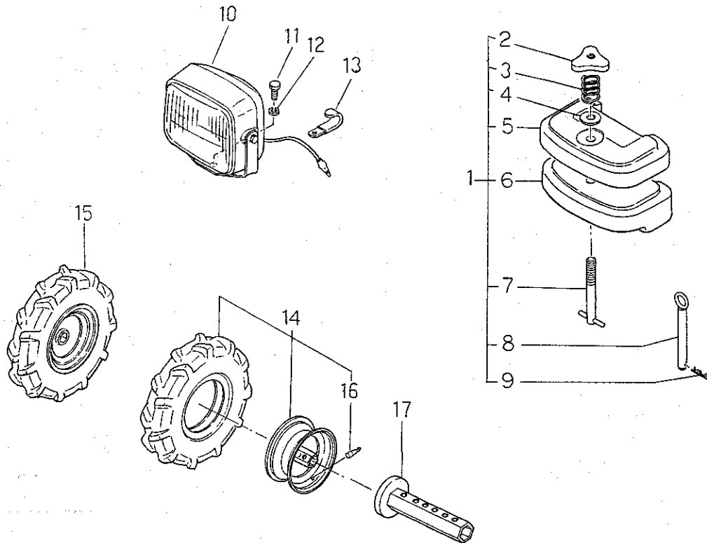
オプション FIG.231 OPTION
