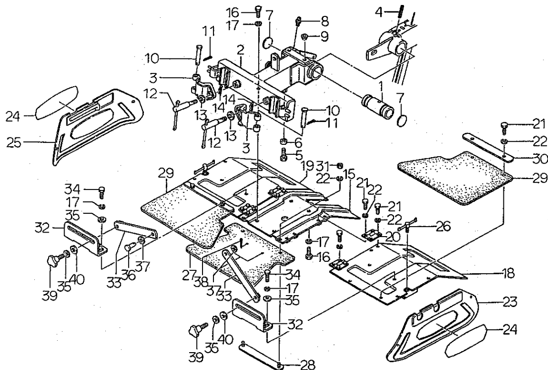
ロータリフレーム, カバー FIG.229 ROTARY FRAME, COVER
