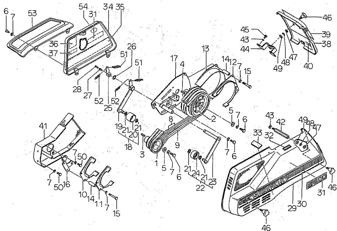
ベルト ドライブ FIG.225 BELT DRIVE
