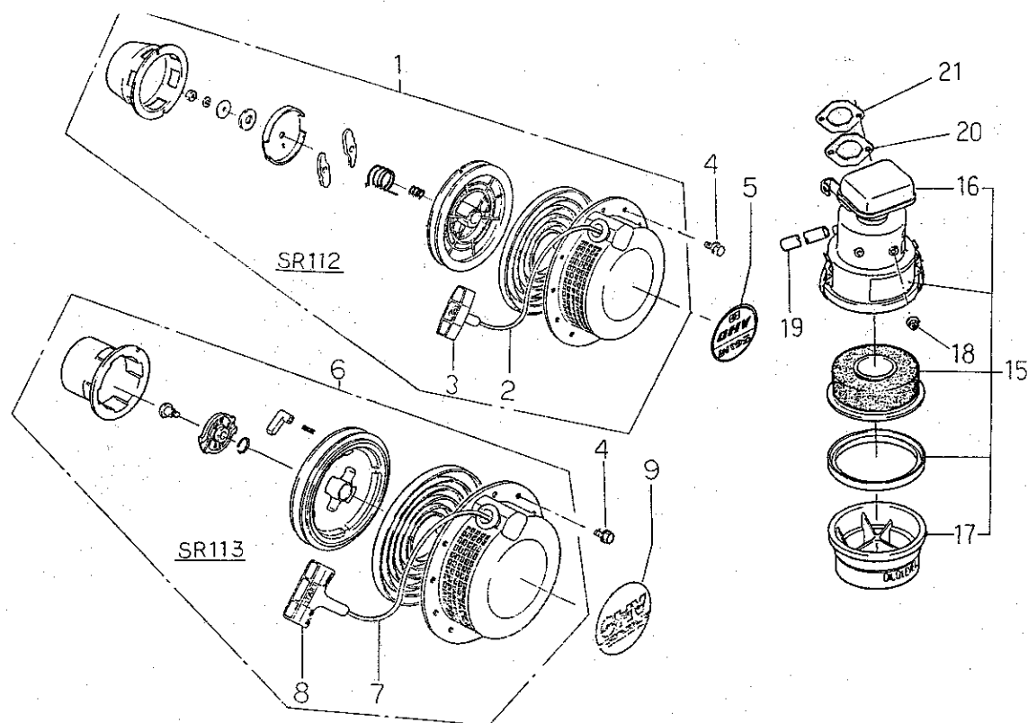
リコイルスタータ,エヤクリーナ FIG.126 RECOIL STARTER, AIR CLEANER
