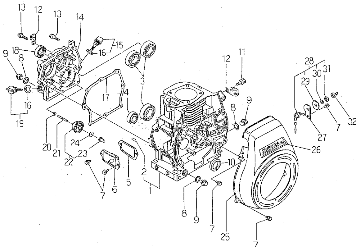
シリンダ ブロック FIG.101 CYLINDER BLOCK
