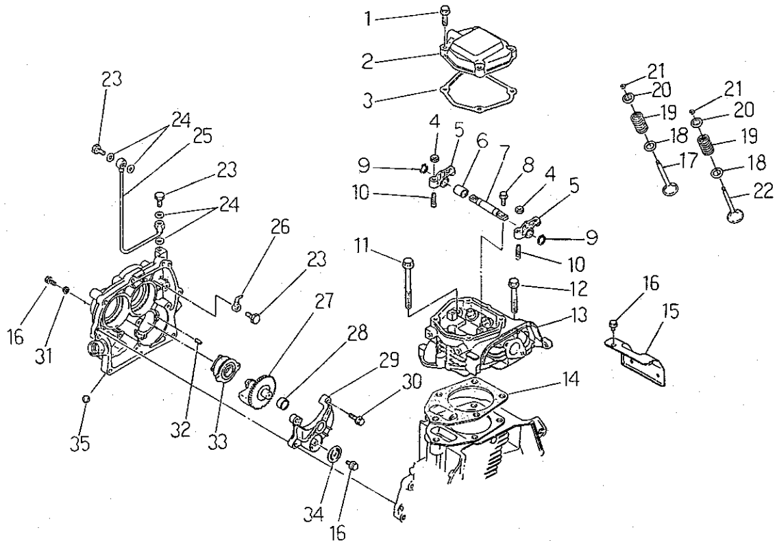
シリカダ ヘッド FIG. 102 CYLINDER HEAD
