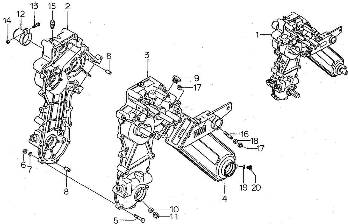
トランスミッション ケース FIG.221 TRANSMISSION CASE
