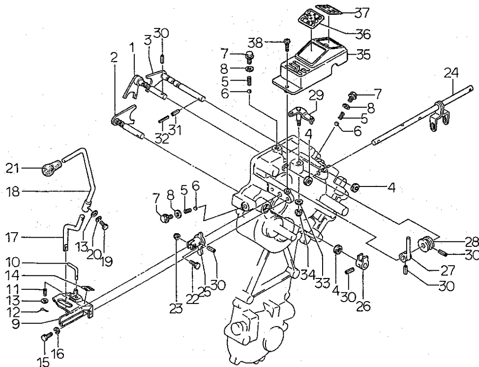
シフタ, チェンジ FIG.224 SHIFTER, CHANGE
