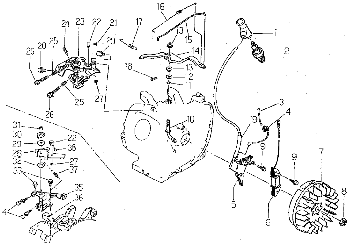
イグニッション, ガバナ FIG.124 IGNITION, GOVERNOR
