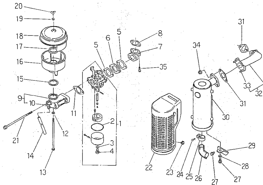
FIG.106 キャブ,エアクリ-ナ,マフラ CARBU, AIR CLEANER, MUFFLER
